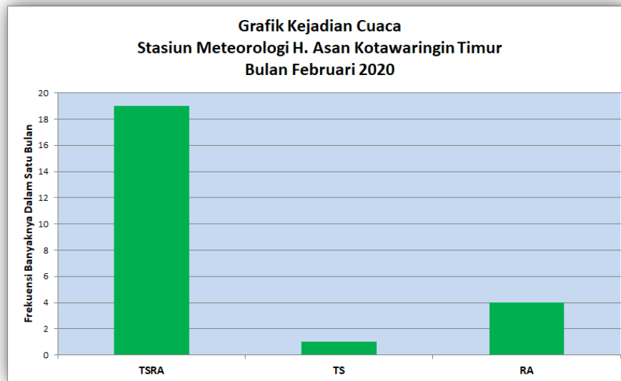
Gambar 9. Grafik Banyak Hari dan Kejadian Cuaca Khusus Bulan Februari 2020
