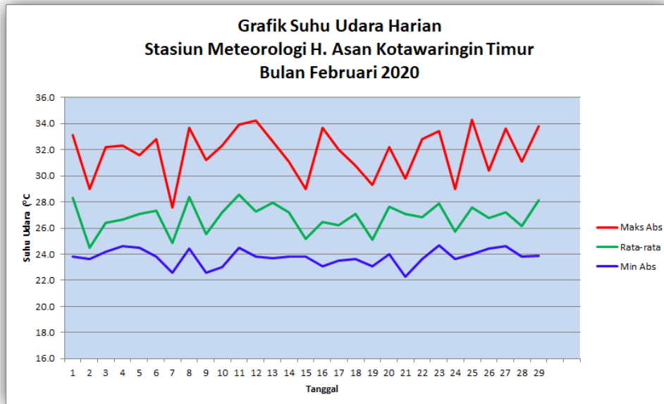
Gambar 2. Grafik Suhu Maksimum dan Suhu Minimum Harian Bulan Februari 2020
