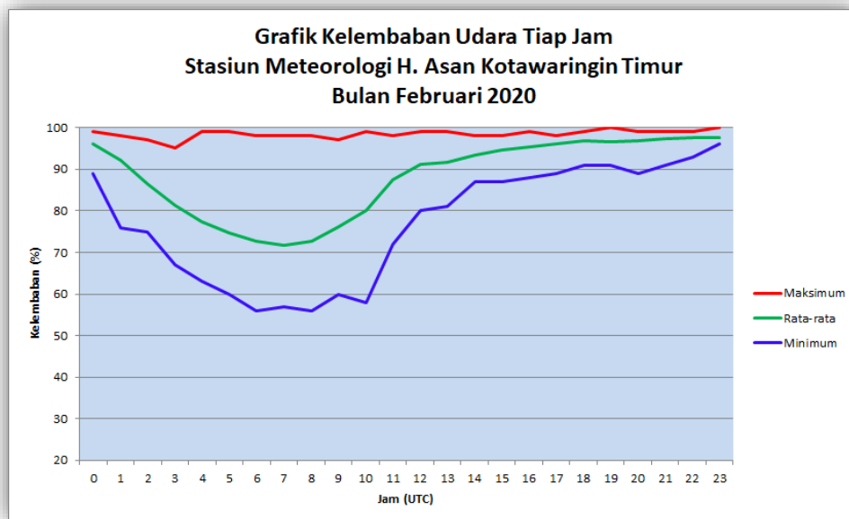
Gambar 3. Grafik Kelembaban Udara Tiap Jam Bulan Februari 2020
