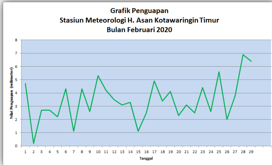
Gambar 5. Grafik Penguapan Harian Bulan Februari 2020
