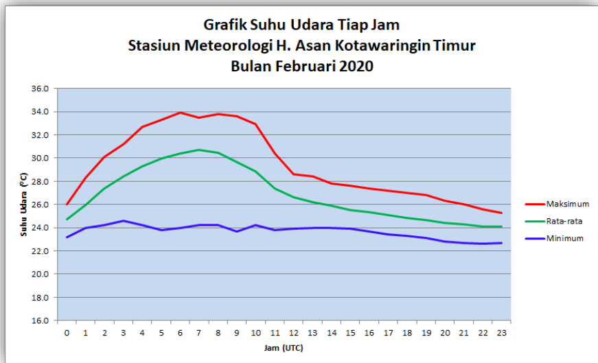
Gambar 1. Grafik Suhu Udara Tiap Jam Bulan Februari 2020
